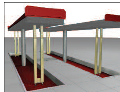
Achsmessstütze
